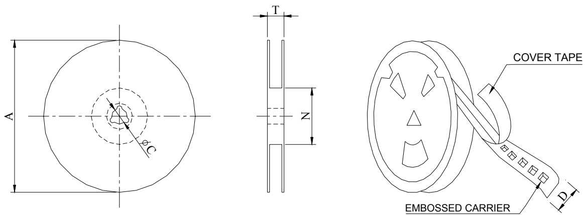
Reel Dimensions
